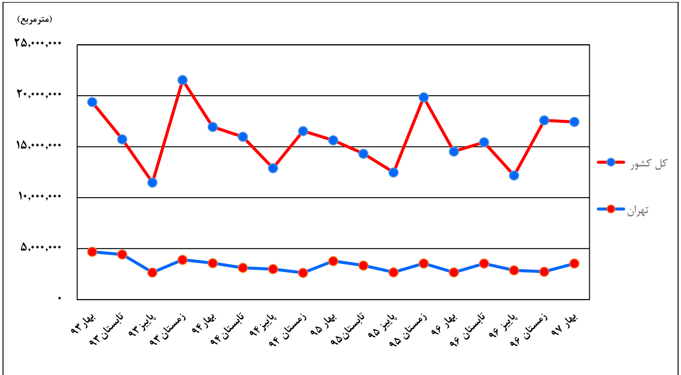
نمودار ۱۱- روند تغییرات مساحت زیربنا در پروانه‌های احداث ساختمانی در شهر تهران و کل کشور از بهار ۱۳۹۳ تا بهار ۱۳۹۷
