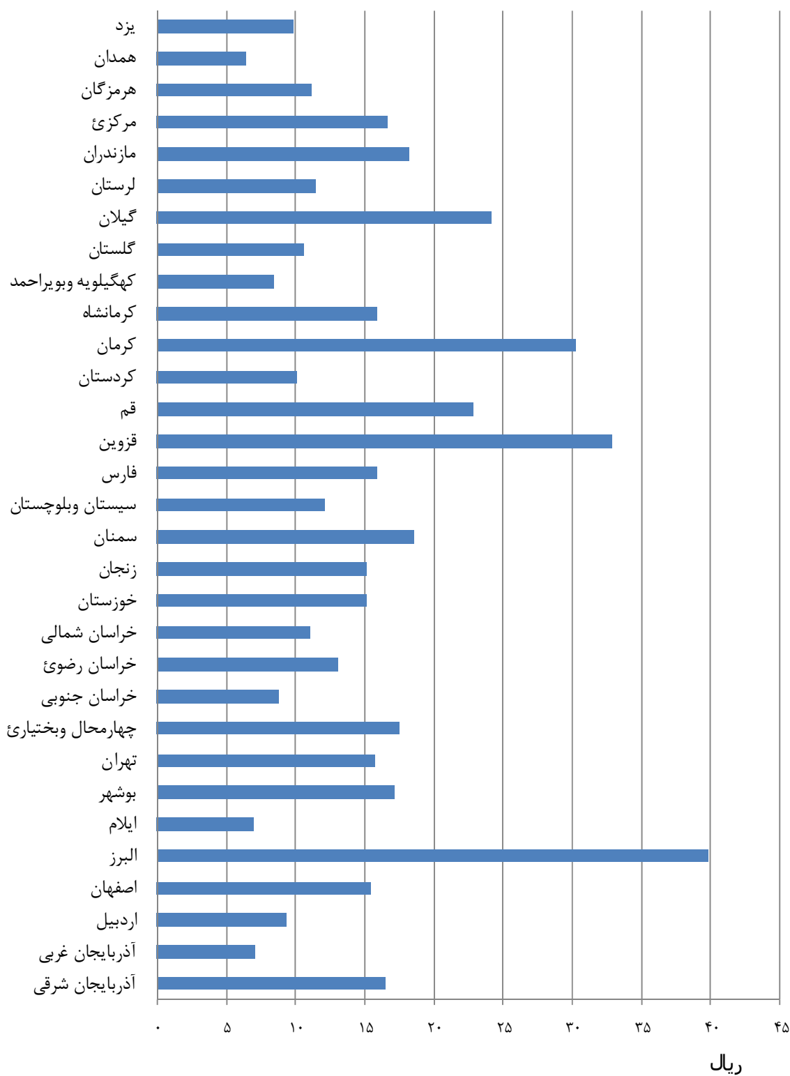
نمودار ۱۴- بهره دهی انرژی در کارگاه‌های صنعتی ۵۰ نفر کارکن و بیش‌تر برحسب استان
